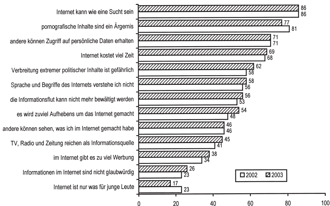
Abb. 5 Offliner: Einstellungen zum Internet 2002 und 2003 trifft voll und ganz/weitgehend zu, in %
